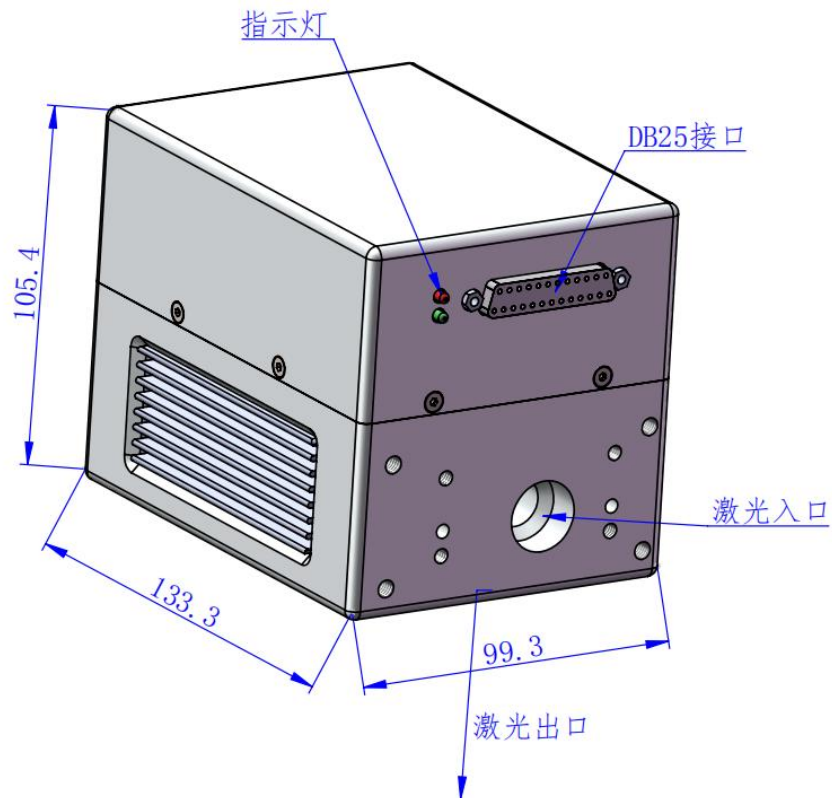
图片 2-1: PROSCAN II 14mm 振镜
