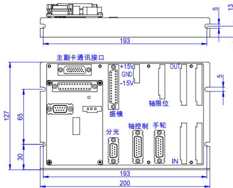
PCIE 副卡
