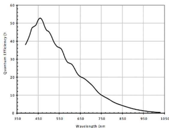
图1-6 LBAS-GE100-07M 响应曲线
