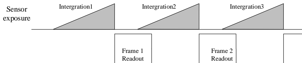
图4-12 内触发模式
