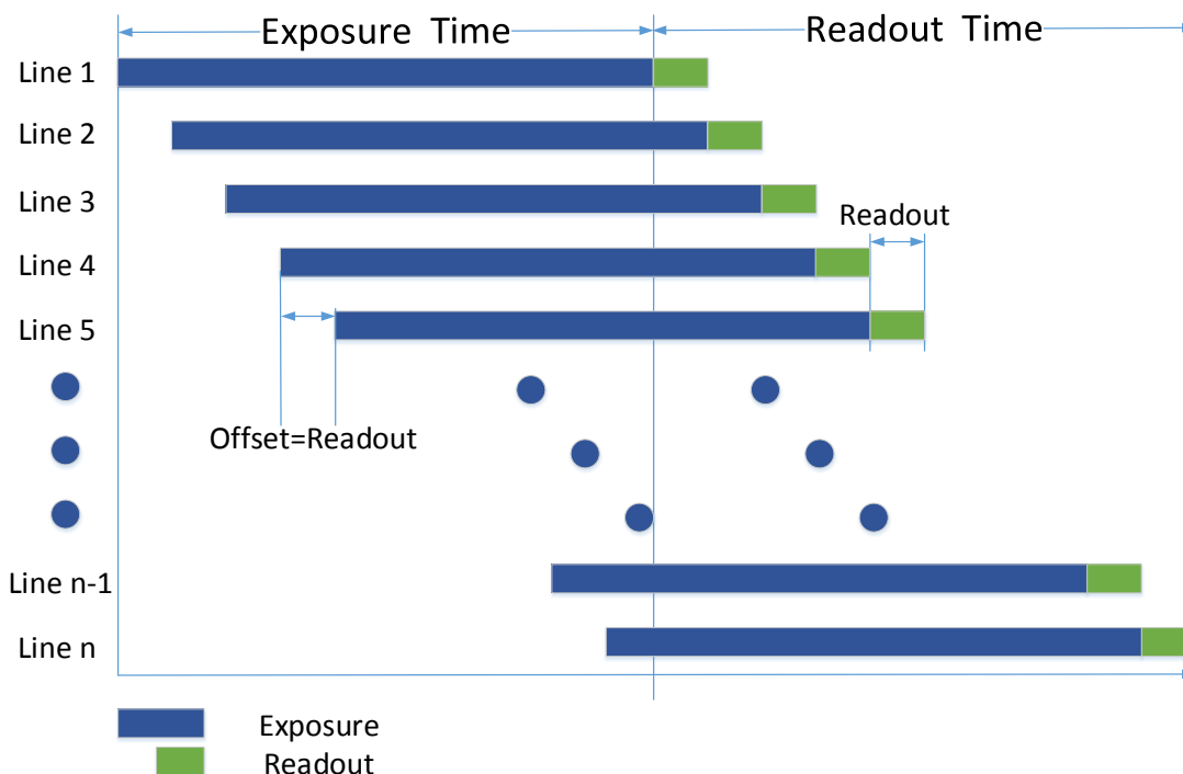
图4-11 卷帘式曝光
