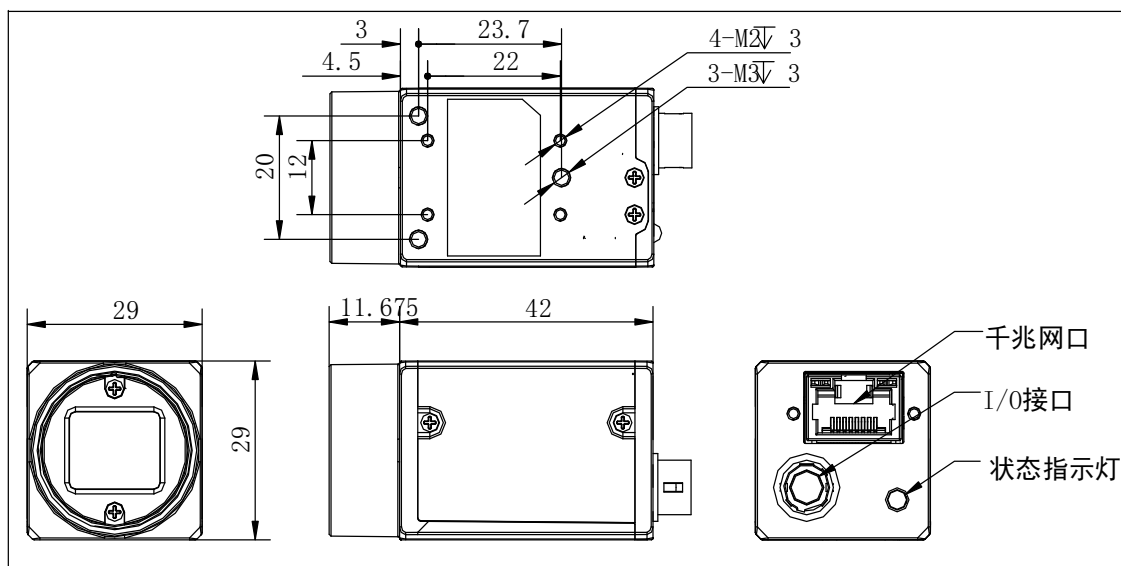
图1-7 相机机械尺寸
