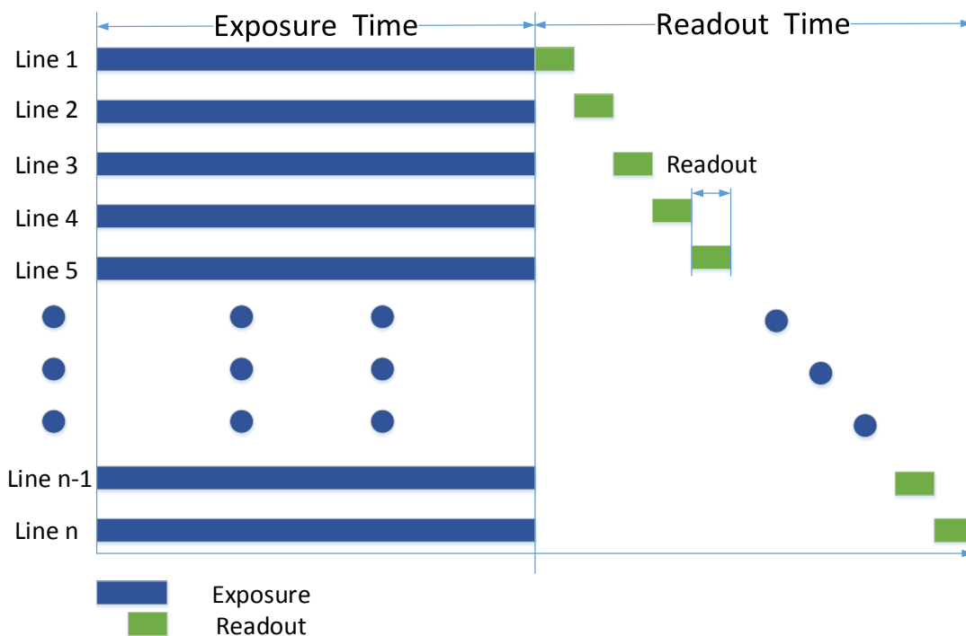
图4-10 全局曝光
