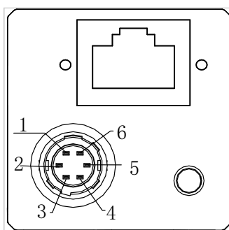
图1-8 相机背面接口
