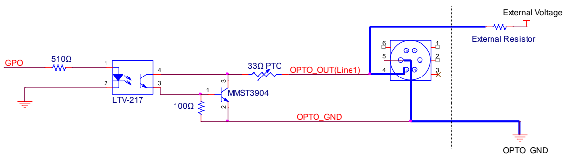
图4-56 输出电路
