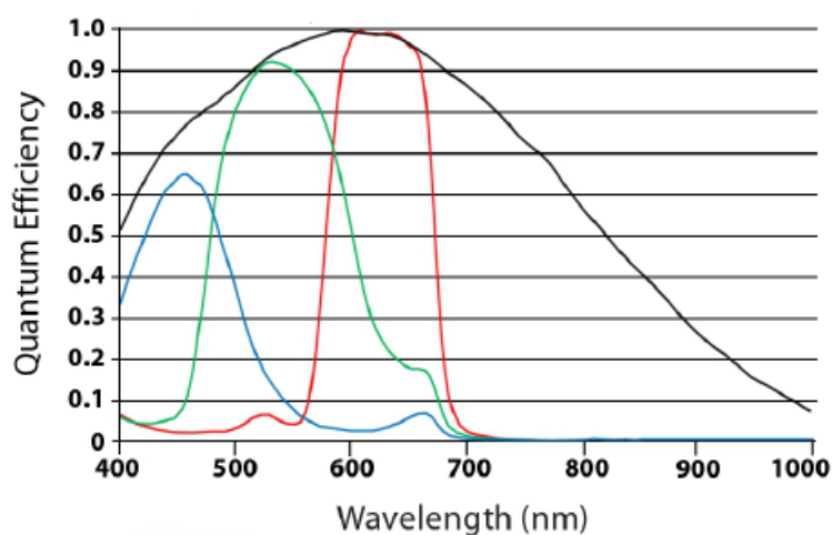
图1-4 LBAS-GE50-23M 响应曲线
