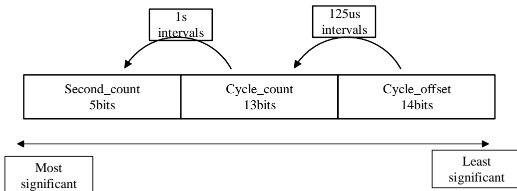
图4-65 时间戳格式
