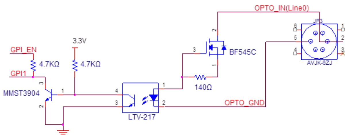
图4-54 输入电路
