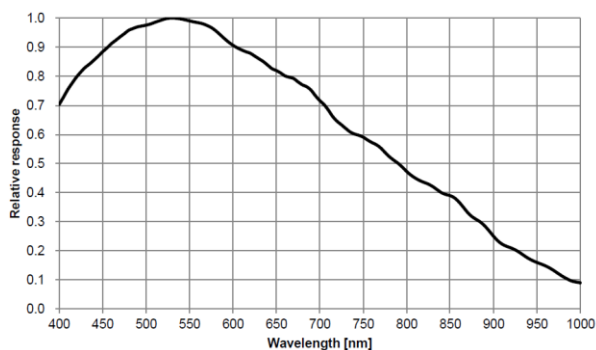
图1-5 LBAS-GE60-17M 响应曲线
