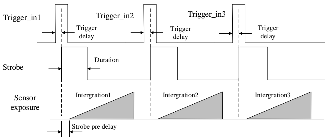
图4-23 Strobe 预输出时序图
