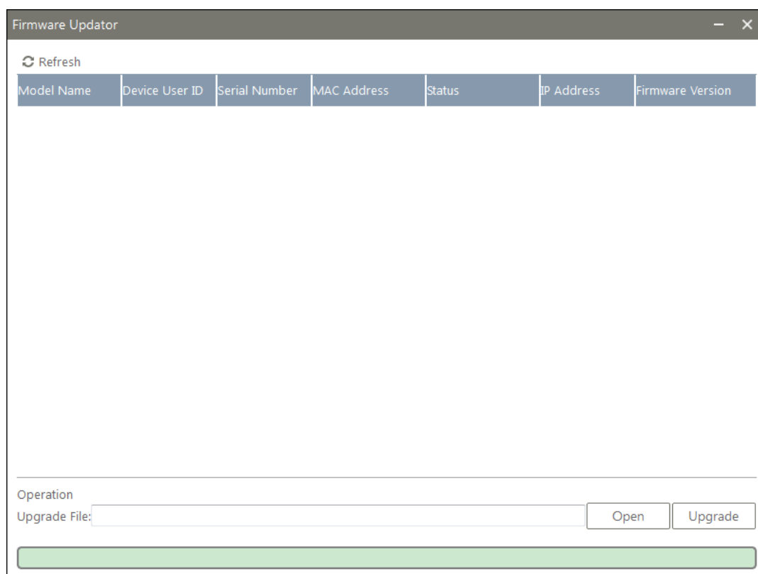
图4-67 固件升级
