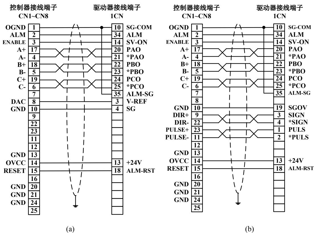
图 6-8 安川 YASKAWA SERVOPACK 系列驱动器速度&力矩控制方式(a)接线/位置控制方式(b)接线
