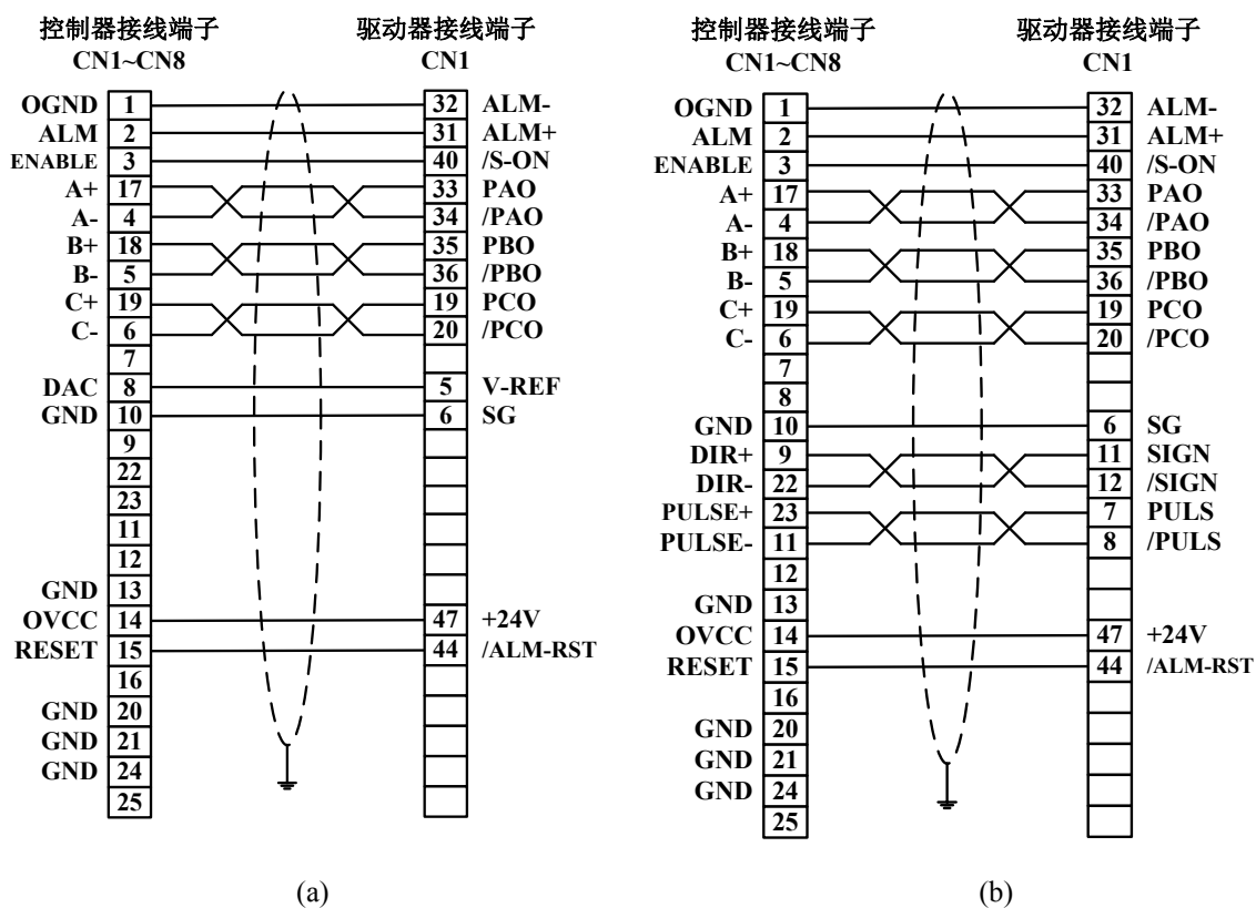
图 6-9 安川 YASKAWA SGDM 系列驱动器速度控制方式(a)/位置控制方式(b)接线
